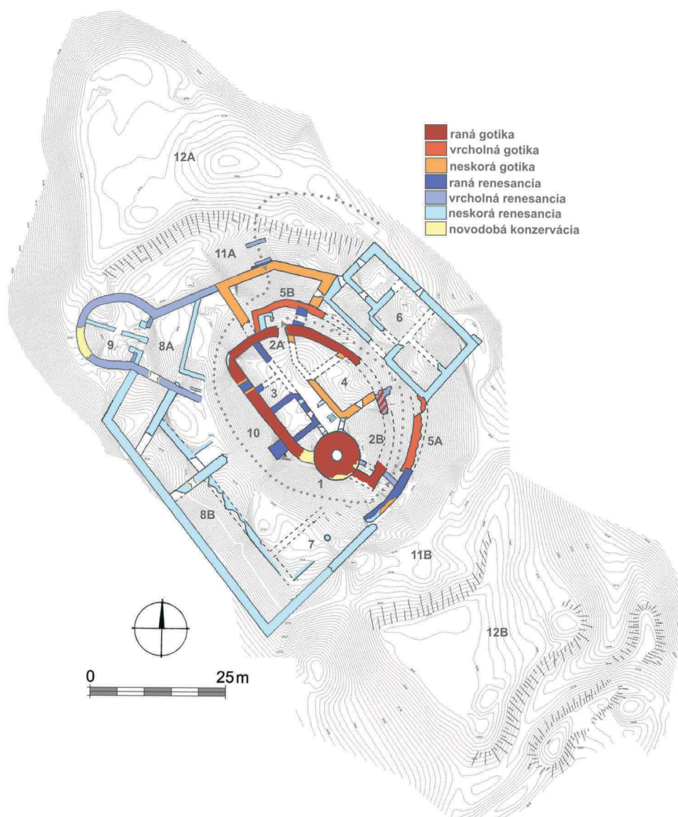
Obr. 2. Pôdorys hradu s vývojovou analýzou. (Analýza a kresba: M. Bóna s využitím výškopisu GEO-CZ a zamerania T. Kozlíka).
